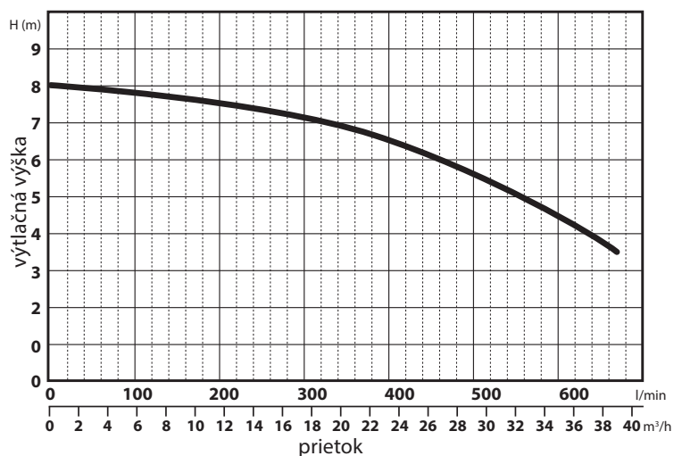
Obr. 1, prietokový graf
