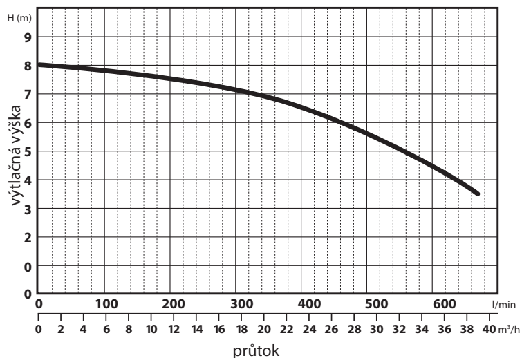
Obr. 1, průtokový graf
